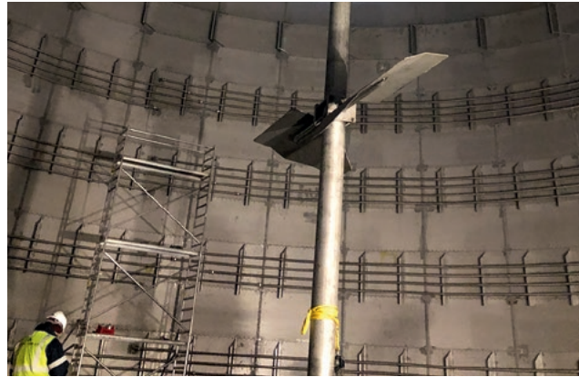
Montage Zentralrührwerk Assembly of central stirring system
