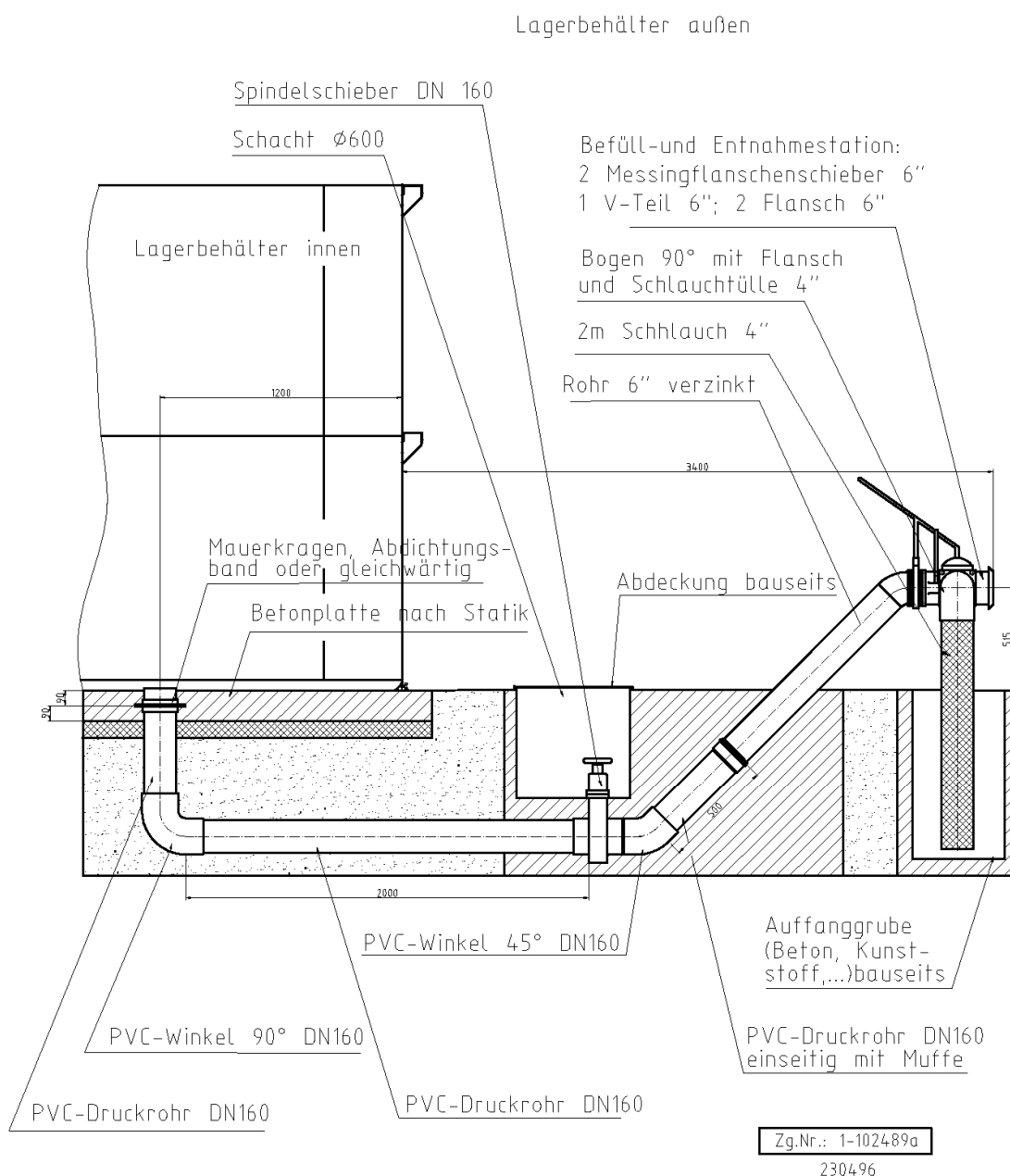
Saug- und Befüllstutzen durch den Behälterboden (Ablafßhahn 6")
