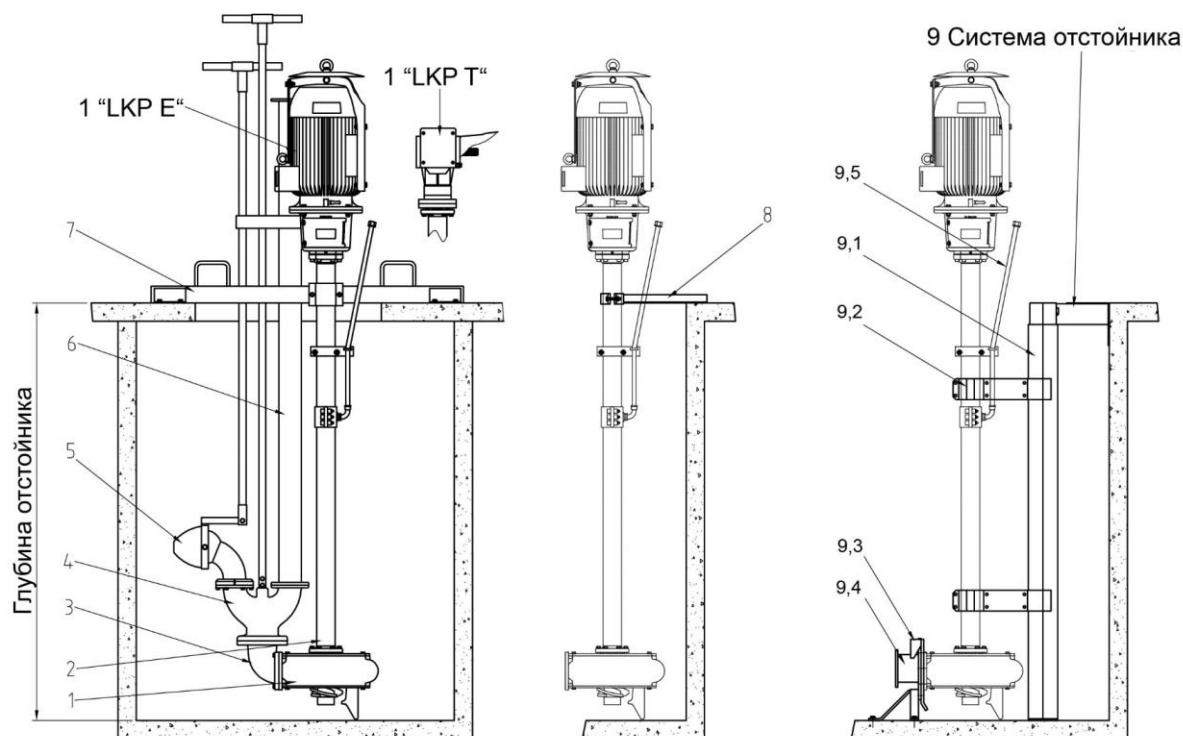
Составные части конструкции с центробежным насосом с длинным валом
