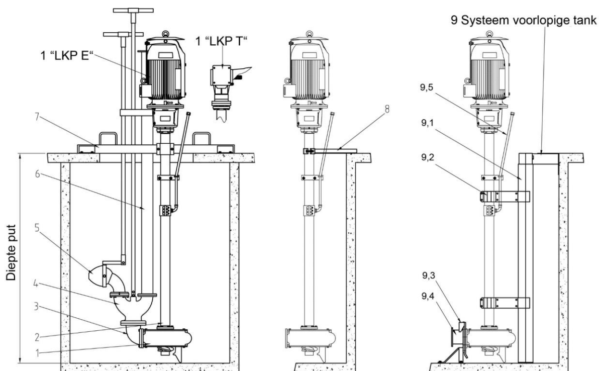
Benaming montageonderdelen voor centrifugaalpompe met lange as
